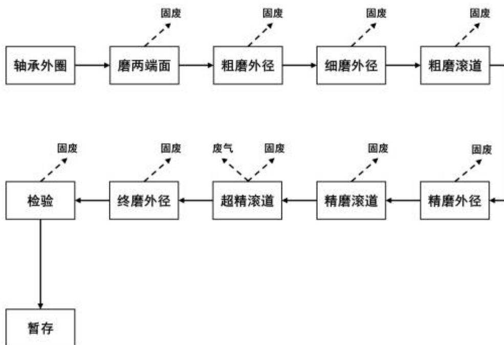
图 2-1 轴承外圈生产工艺流程及产污节点图
