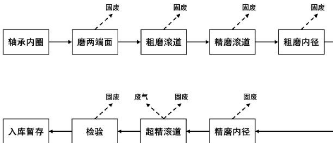
图 2-2 轴承内圈生产工艺流程及产污节点图
