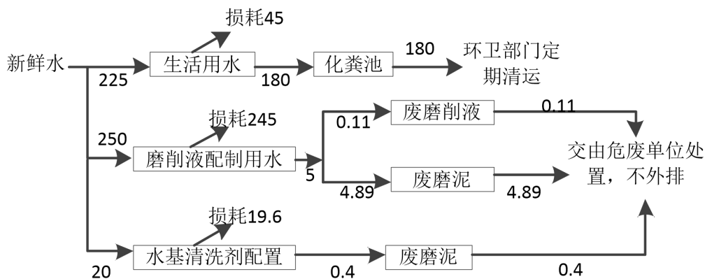
图 2-2 该项目水平衡示意图 (m 3 /a)
