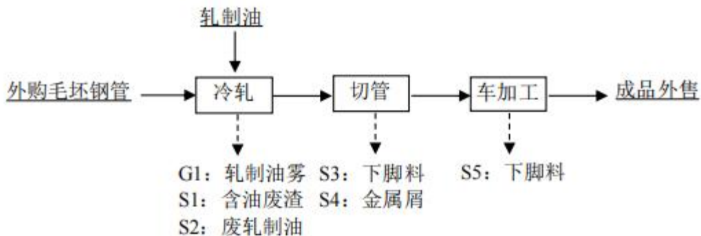
图 2-1 生产工艺流程及产污节点图
